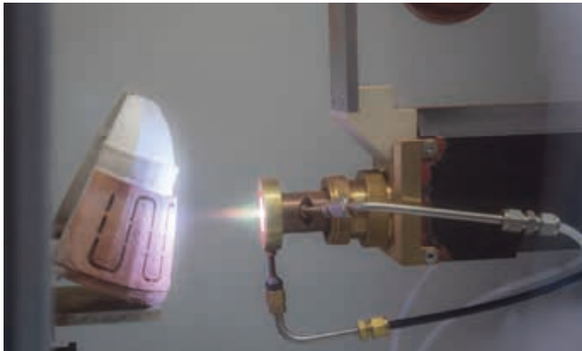
Experimentelle Plasmabeschichtung von Kunststoffen
